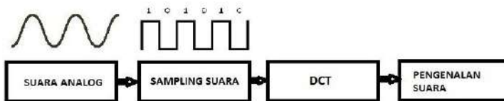
Gambar 6 Skema sistem pengujian hafalan Al Qur’an
