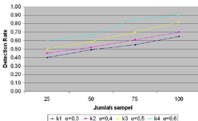
Gambar 8 Grafik unjuk kerja transformasi Kosinus terhadap sistem pengujian hafalan Al Qur'an (k_1) , (k_2) , (k_3) , dan (k_4) .
