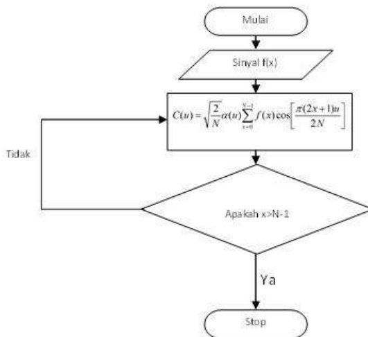
Gambar 7 Diagram alir transformasi Kosinus
