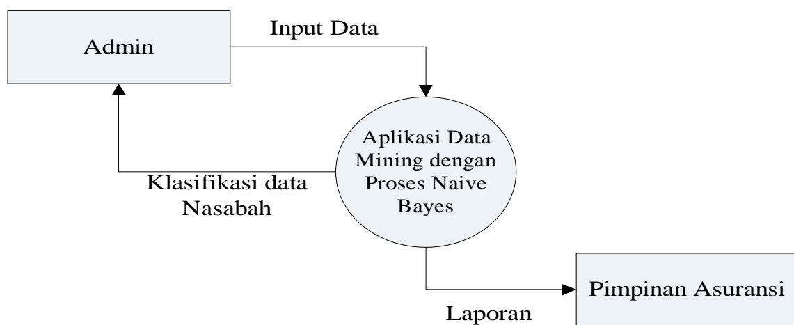
Gambar 4. Diagram Konteks
