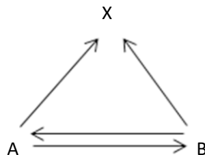
Gambar 1. segitiga ABX
