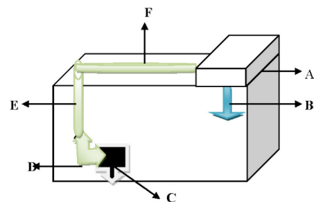
Gambar 1. Desain media filter. A: tempat penempatan bahan filter ijuk, jerami padi dan ampas tebu, B: selang pengeluaran air hasil filter, C: mesin pengisap air, D, E, F: selang pengisap air.
